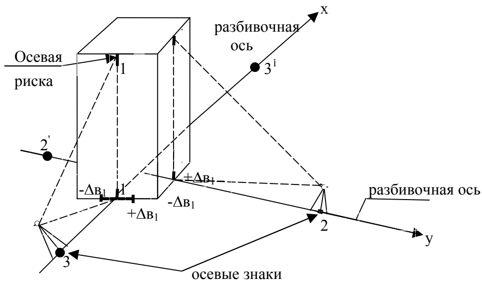
Рисунок 38 – Схема выверки вертикальности колонны методом наклонного проектирования
