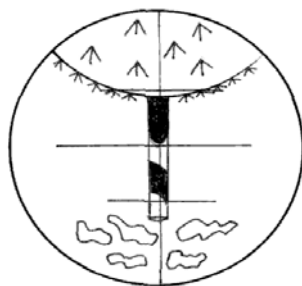
Рисунок 9 – Наведение перекрестия сетки нитей на съёмочную точку
