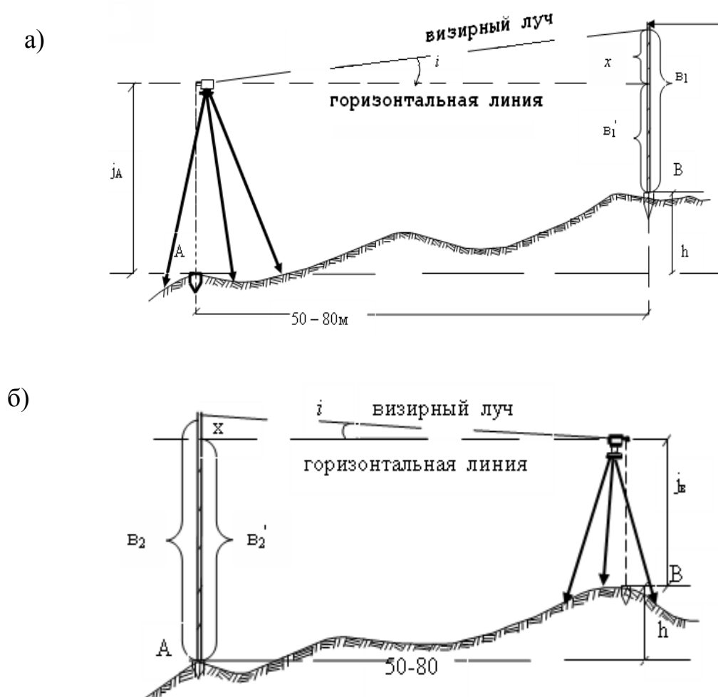
Рисунок 18 а,б - Проверка основного геометрического условия нивелира
