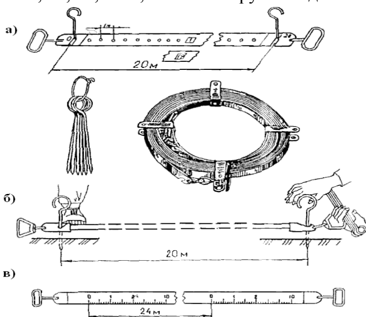
Рисунок 3а, б, в – Мерные ленты
