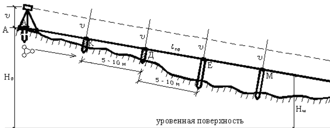
Рисунок 28 – Схема выноса линии с заданным проектным уклоном
