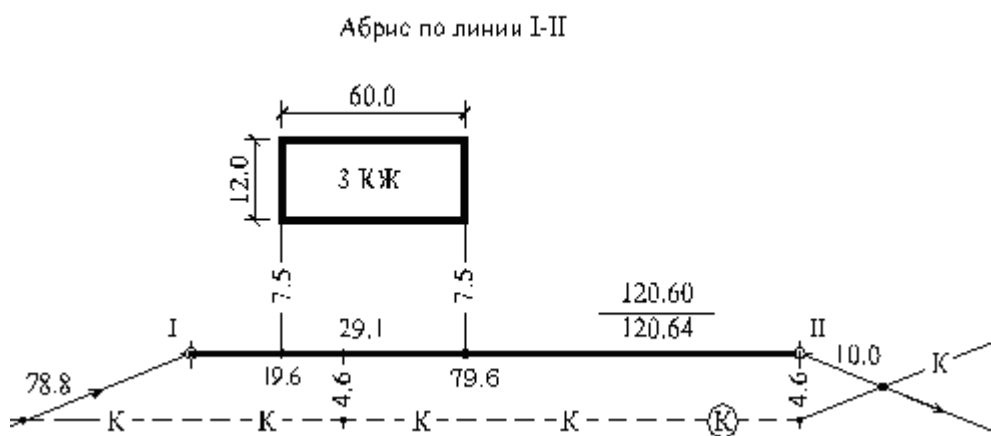
Рисунок 14 – Способ прямоугольных координат
